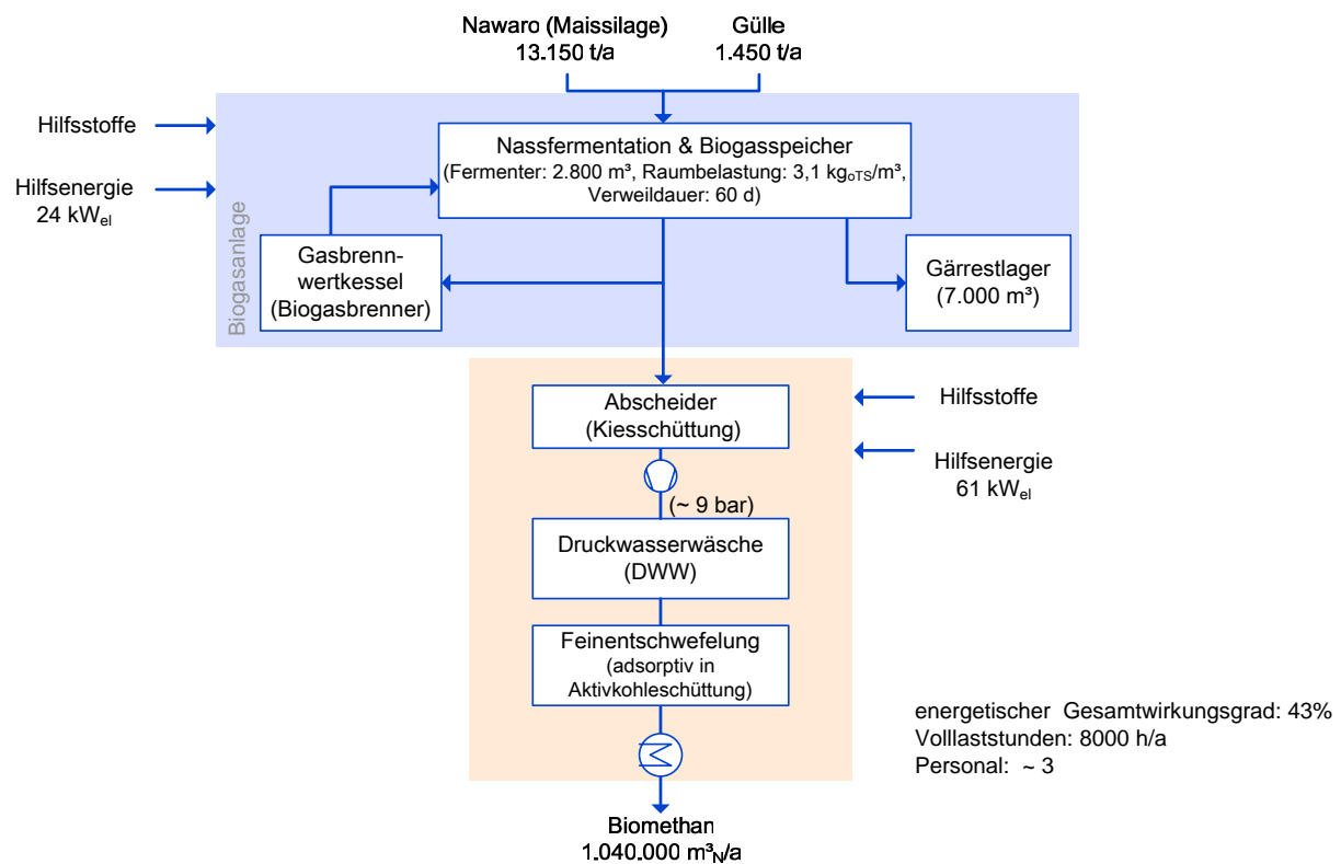
Abbildung 2-6: Referenzkonzept „Biomethan aus Biogas“ – 1,3 MW th -Anlage /2/
