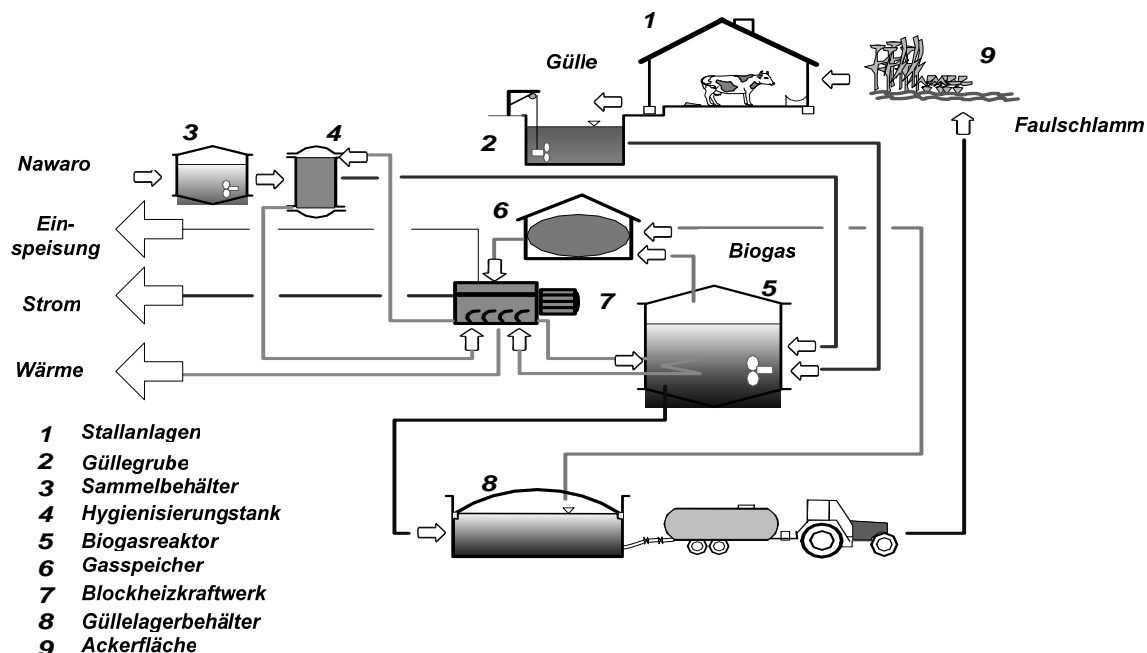
Abbildung 2-3: Schema einer landwirtschaftlichen Biogasanlage mit Verwendung von Kosubstraten /7/
