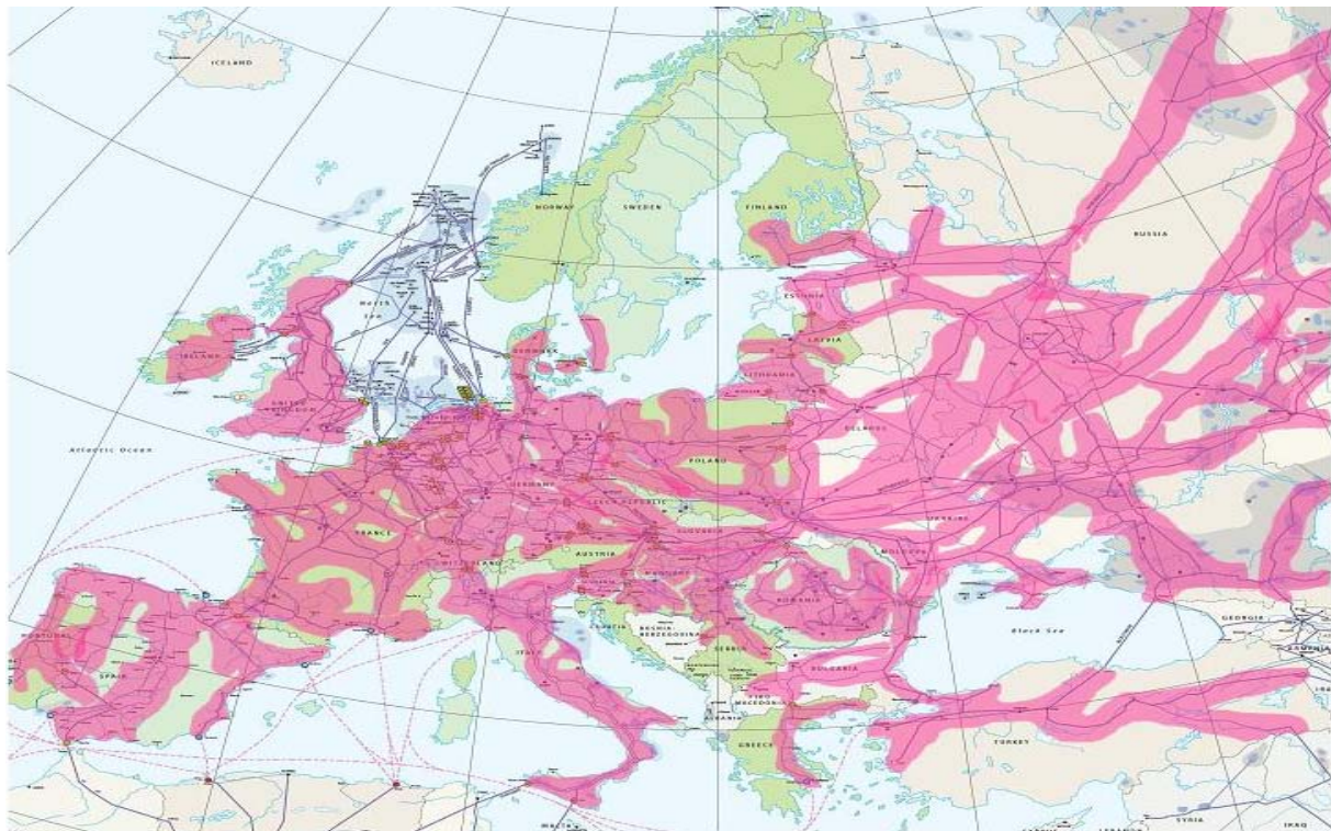
Abbildung 3-3: Einzugsgebiete für Bio-SNG-Anlagen
