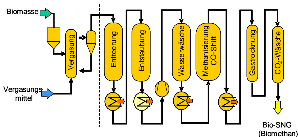
Abbildung 2-5: Verfahrensprinzip zur Herstellung von Bio-SNG (Biomethan), nach /36/
