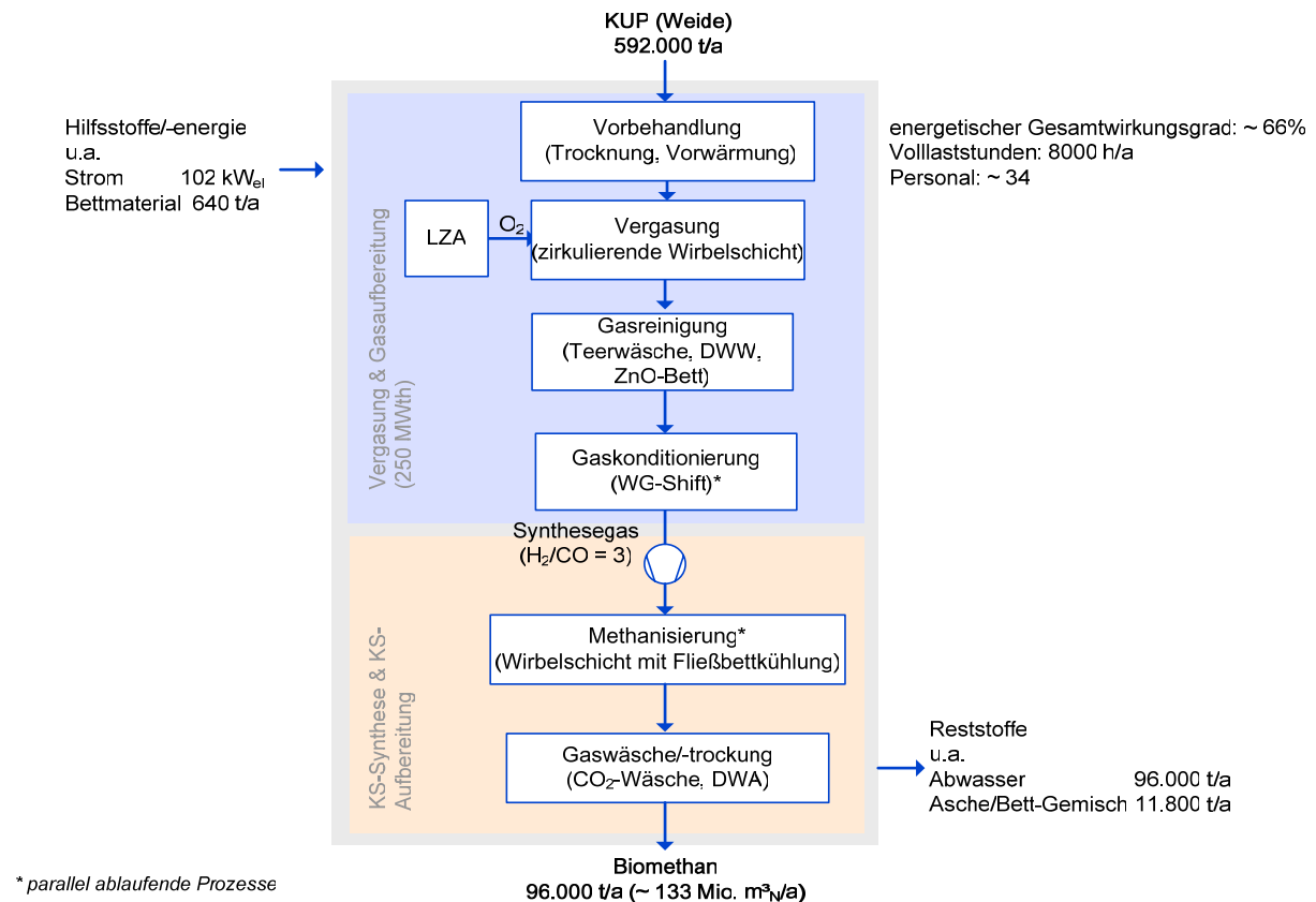
Abbildung 2-7: Referenzkonzept „Biomethan aus Bio-SNG“ – 167 MW th -Anlage /2/
