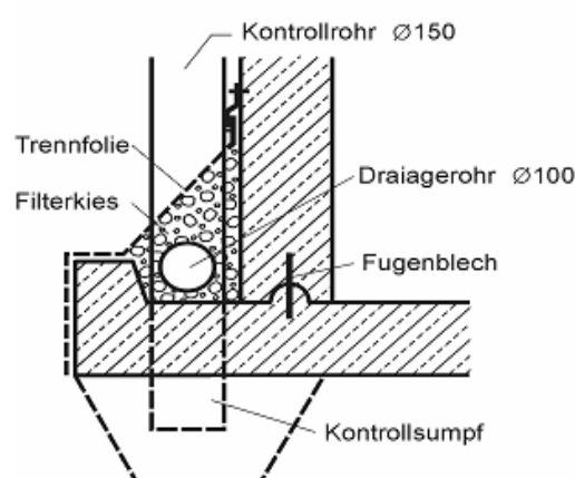
Abb. 14: Alternative zur Dichtungsbahn
