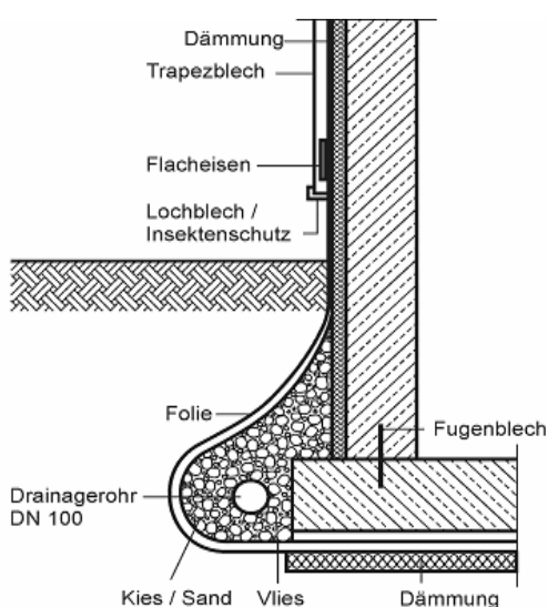
Abb. 13: Dichtungsbahn
