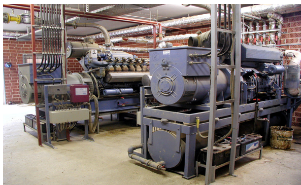
Abb. 7: BHKW ohne Wanne – (Fußboden ist entsprechend herzustellen)
